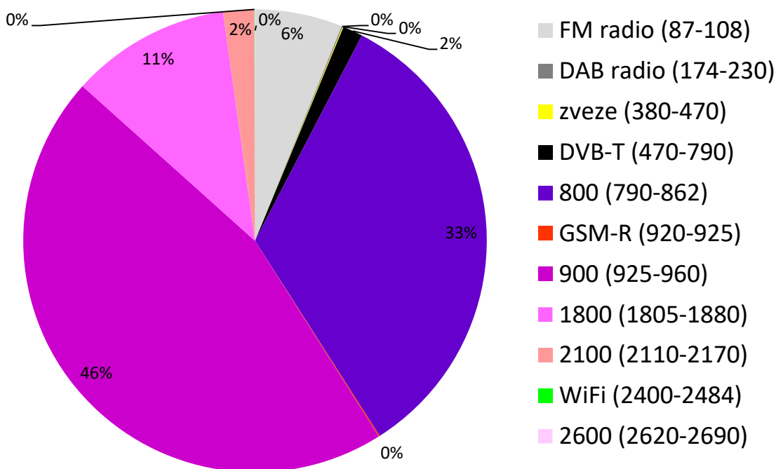
S 18: Prispevek posameznih frekvenčnih območij k skupnim povprečnim sevalnim obremenitvam za podeželje.
