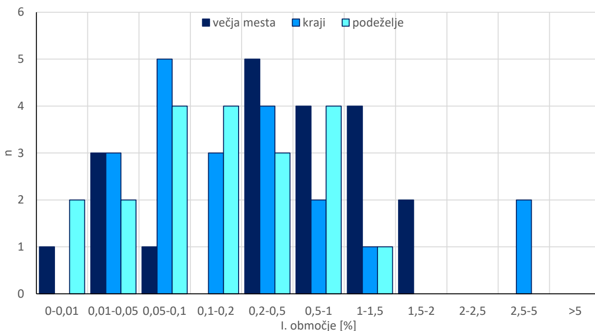
S 10: Histogram povprečnih vrednosti sevalnih obremenitev v odstotkih mejnih vrednosti za I. območje varstva za različne tipe okolja (večja mesta, kraji, podeželje) za frekvenčno območje 900 MHz.
