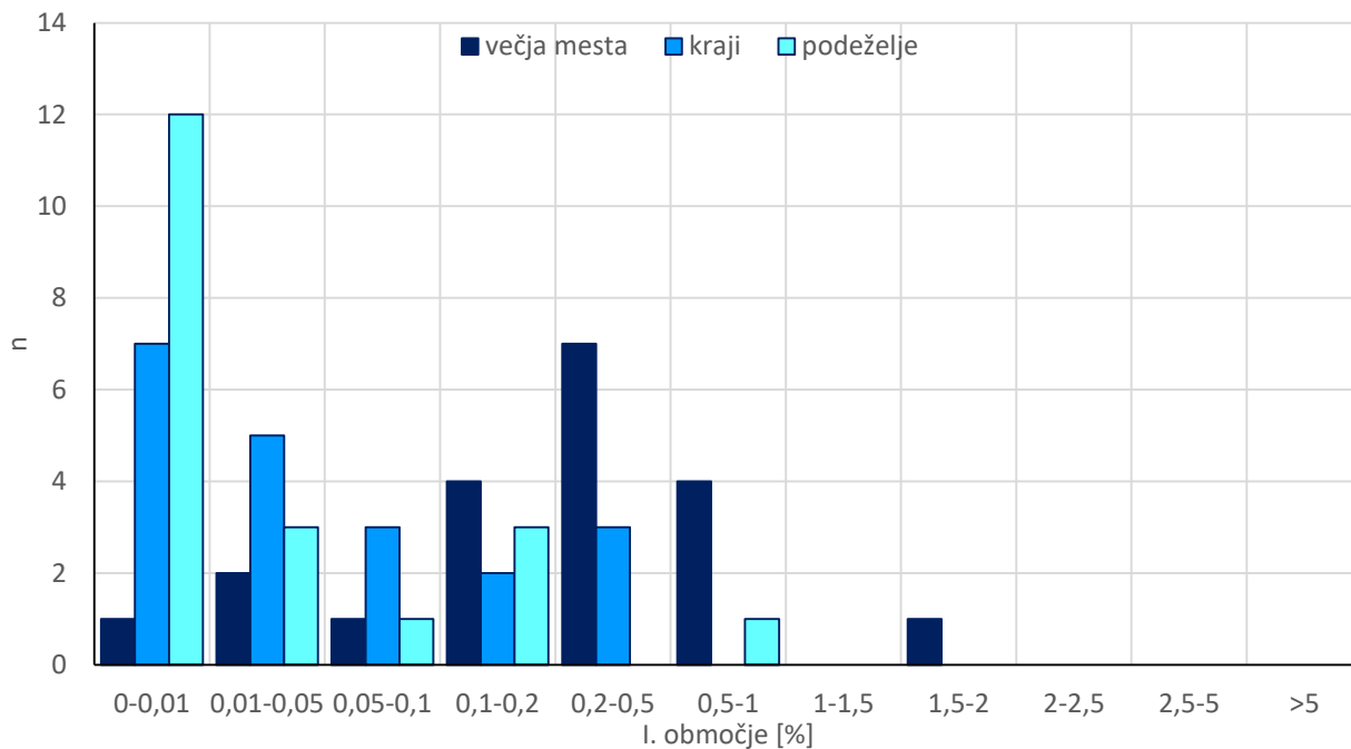
S 12: Histogram povprečnih vrednosti sevalnih obremenitev v odstotkih mejnih vrednosti za I. območje varstva za različne tipe okolja (večja mesta, kraji, podeželje) za frekvenčno območje 1800 MHz.
